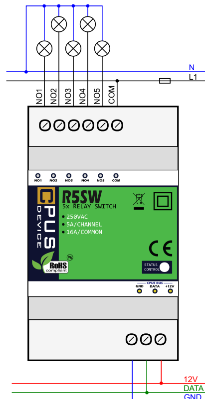
Obr. 3 - Príklad zapojenia R5SW-1A
